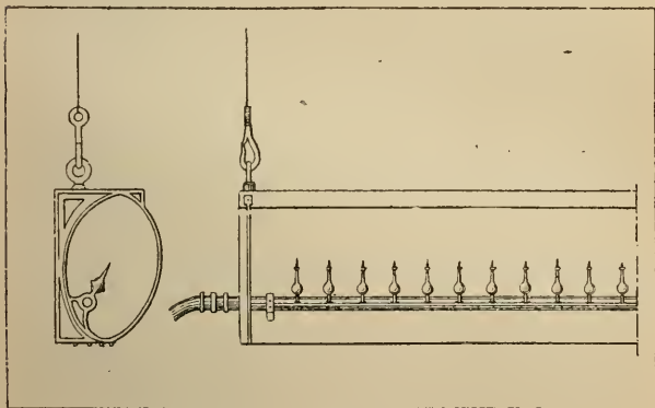
Fig. 23. — Détail d'une herse.
